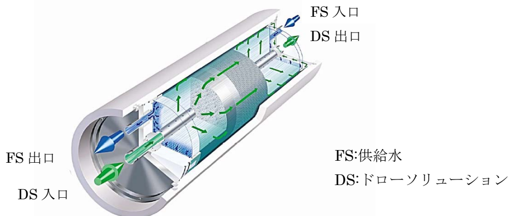
「正浸透用大型中空糸膜モジュール (イラスト図)」
