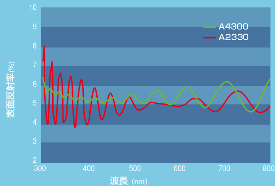
HC塗工後の反射スペクトル (原反厚み125 \mu m)
