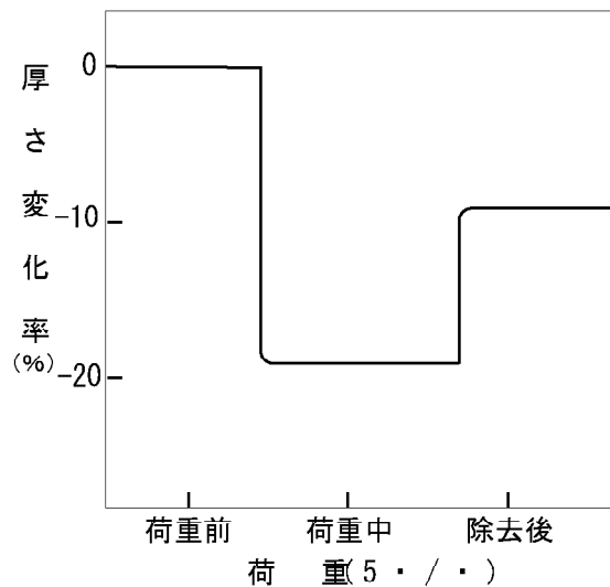
クッション性 (圧縮率と回復率)
