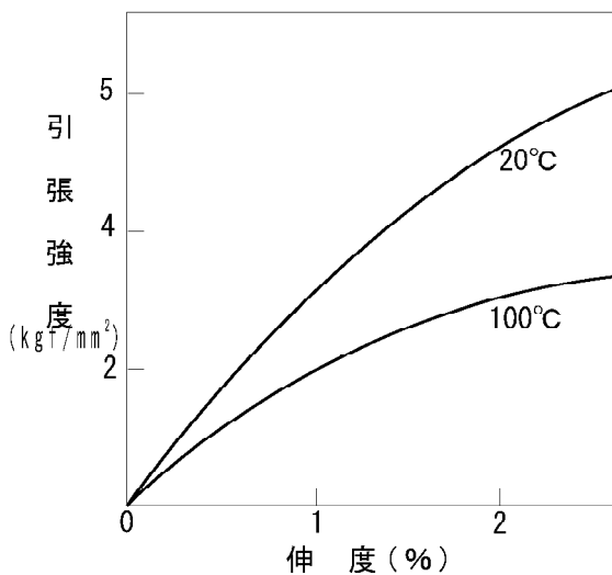
温度と引張強伸度
