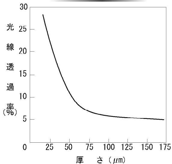
厚みと光線透過率
