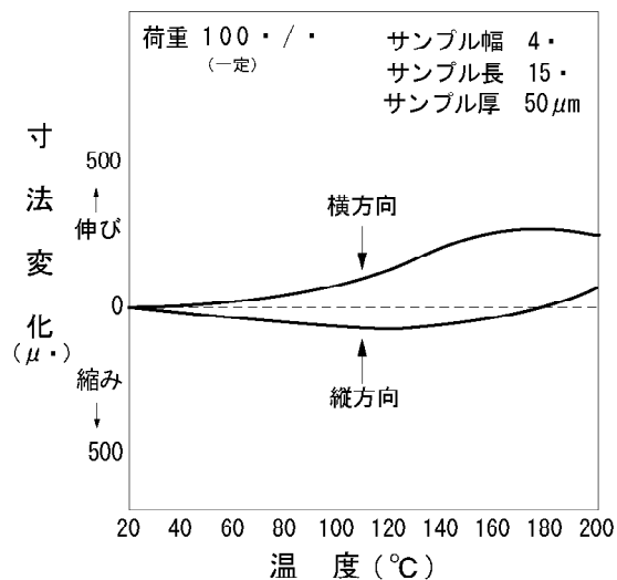
温度と寸法変化
